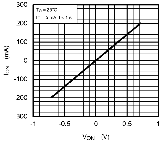
Fig. 12.4 I_{ON} - V_{ON}
